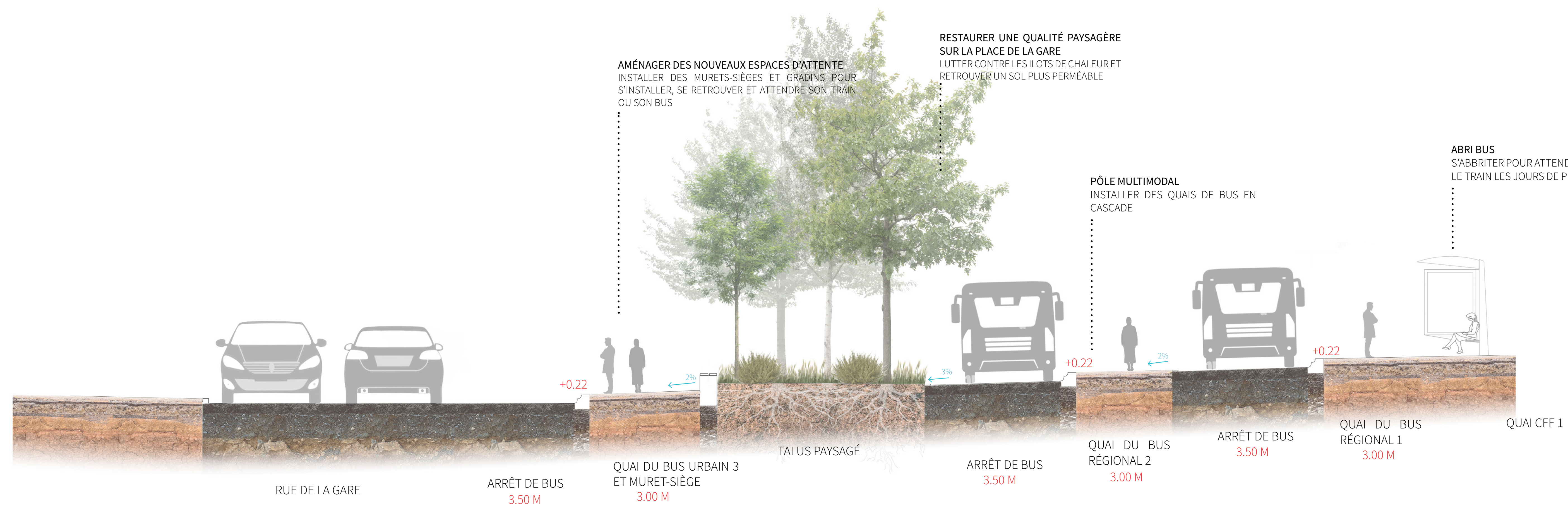
COUPE A-A' UN PÔLE MULTIMODAL EN CASCADE
